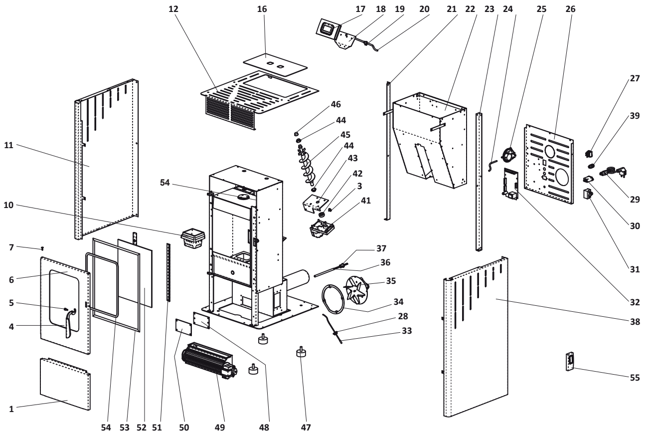
Abb. 14 Explosionszeichnung
