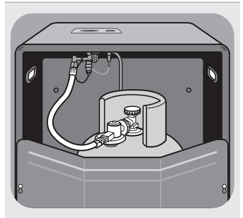
Abb.3: Installation der Gasflasche (Abb. modellabhängig)
