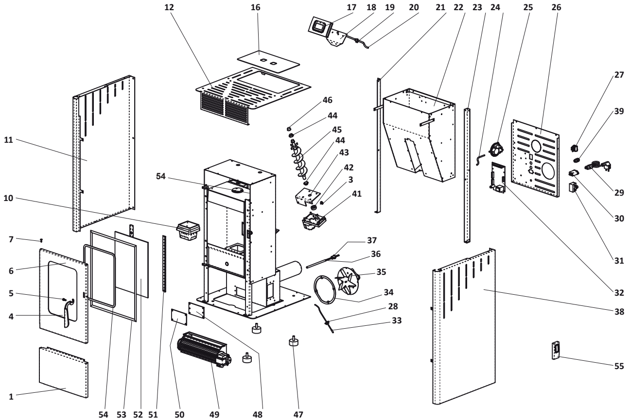
Abb. 14 Explosionszeichnung
