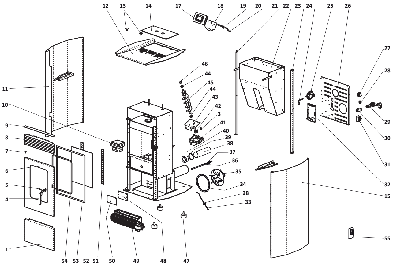
Abb. 14 Explosionszeichnung
