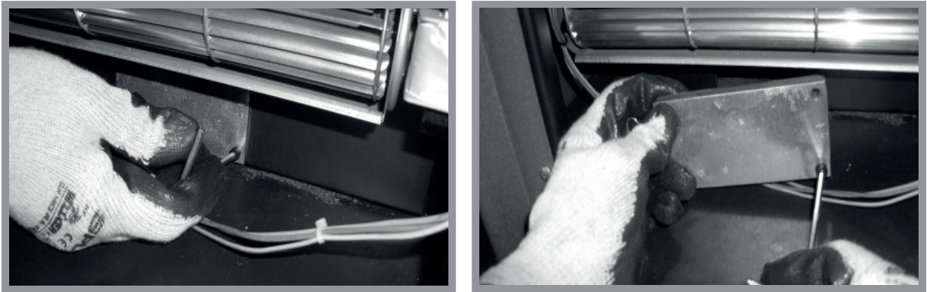
Abb. 13b: Aufschrauben der inneren Abdeckplatte
