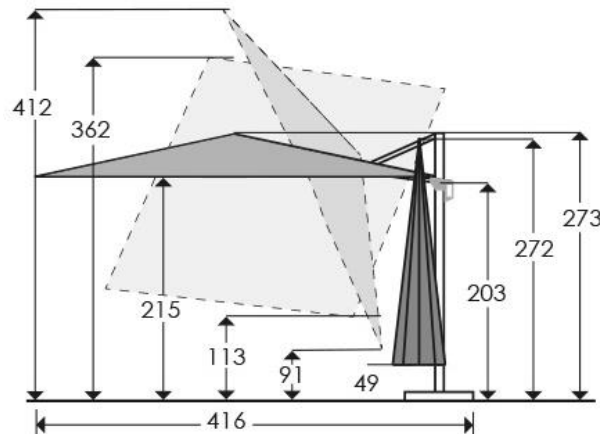
Διαστάσεις (cm)
